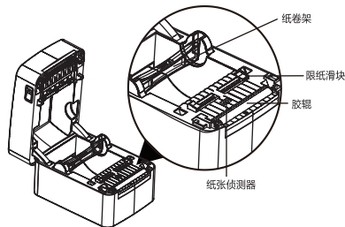
纸卷架
